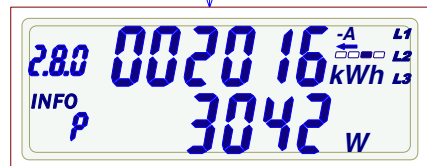
Abb. 8: Anzeige 2- Richtungszähler
