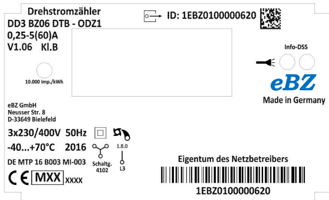
Abb. 4: Leistungsschild des DD3 (Beispiel)
