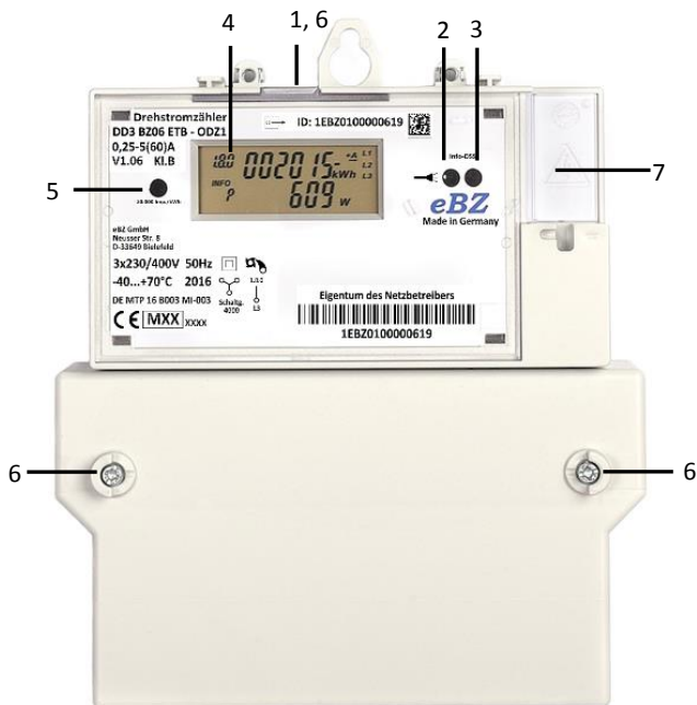
Abb. 1: Merkmale des Zählers DD3
