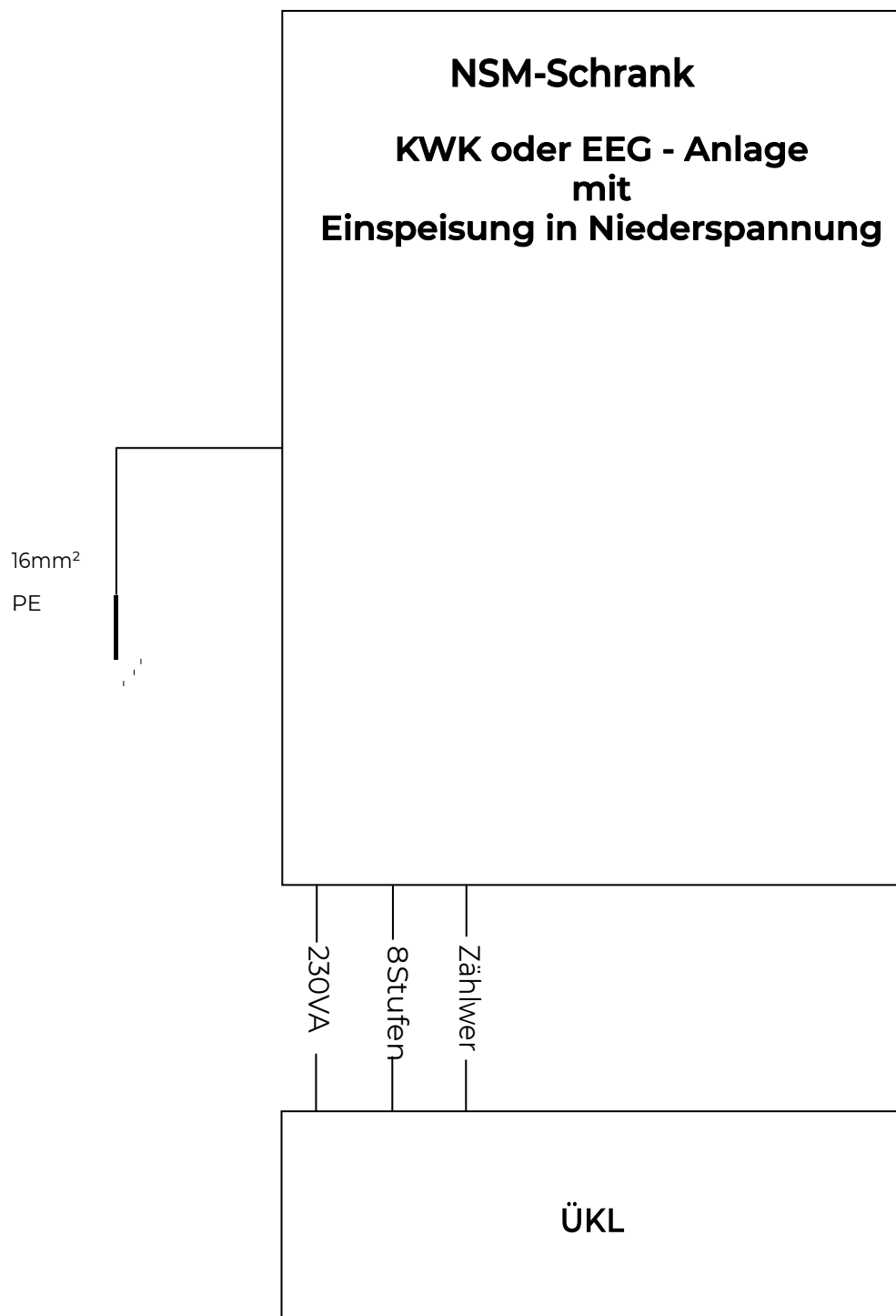
Schema 1: KWK oder EEG Anlagen größer 100 kW mit Einspeisung in die Niederspannung
